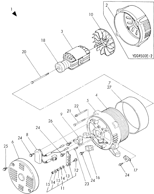
Fig.45 GENERATOR
