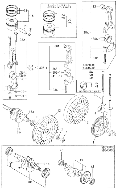
Fig. 94 CRANKSHAFT / PISTON / ROD
