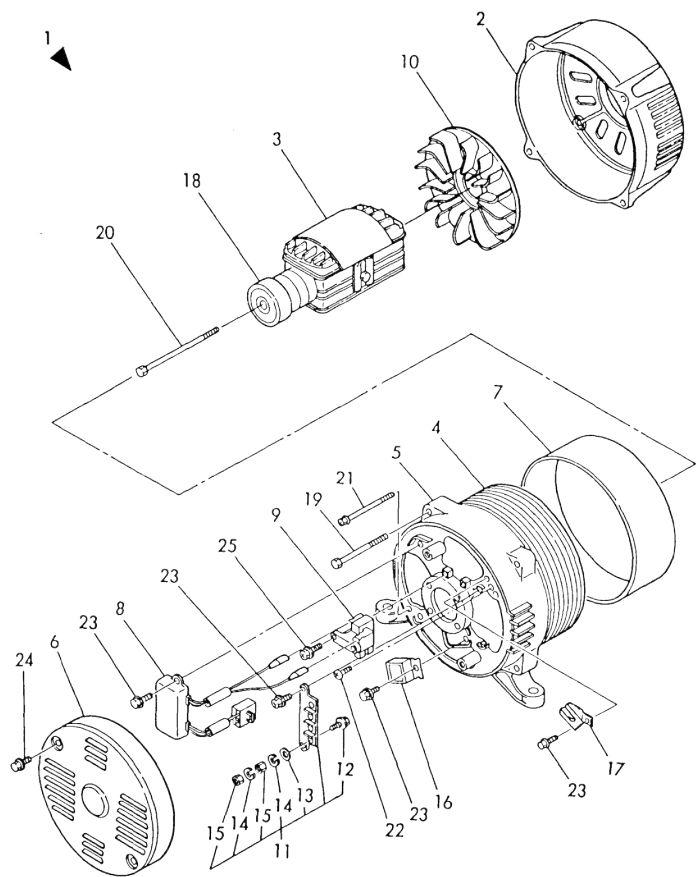
Fig. 120 GENERATOR
