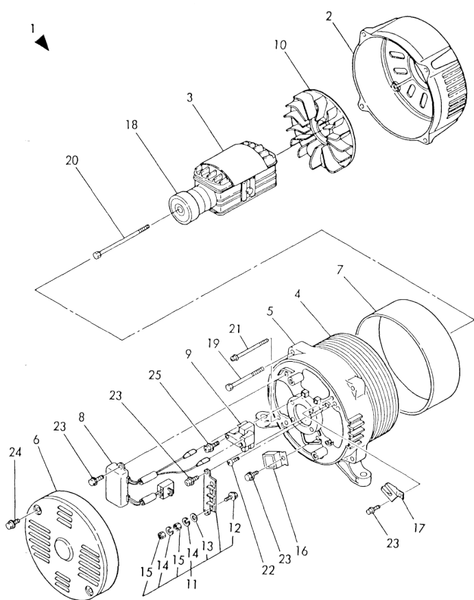
Fig. 104 GENERATOR
