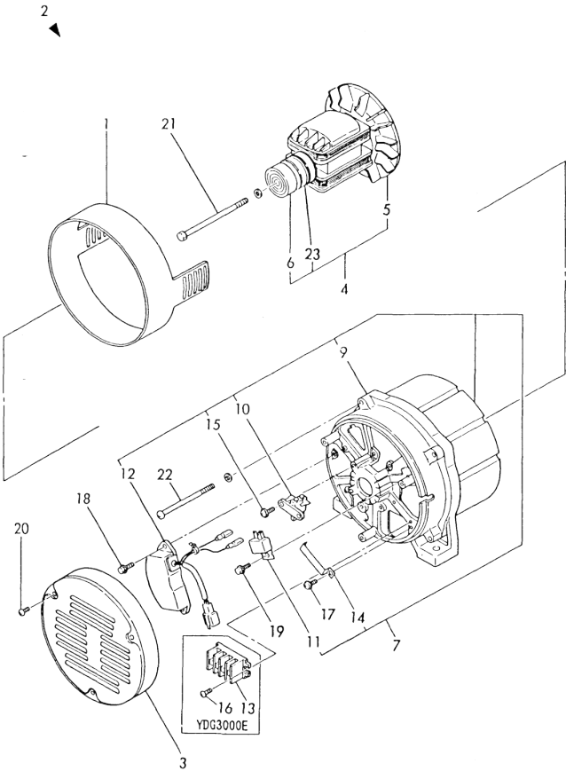
Fig. 119 GENERATOR
