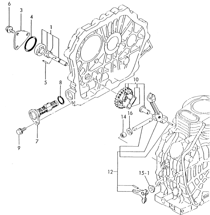
Fig.95 L. O. DEVICE & GOVERNOR
