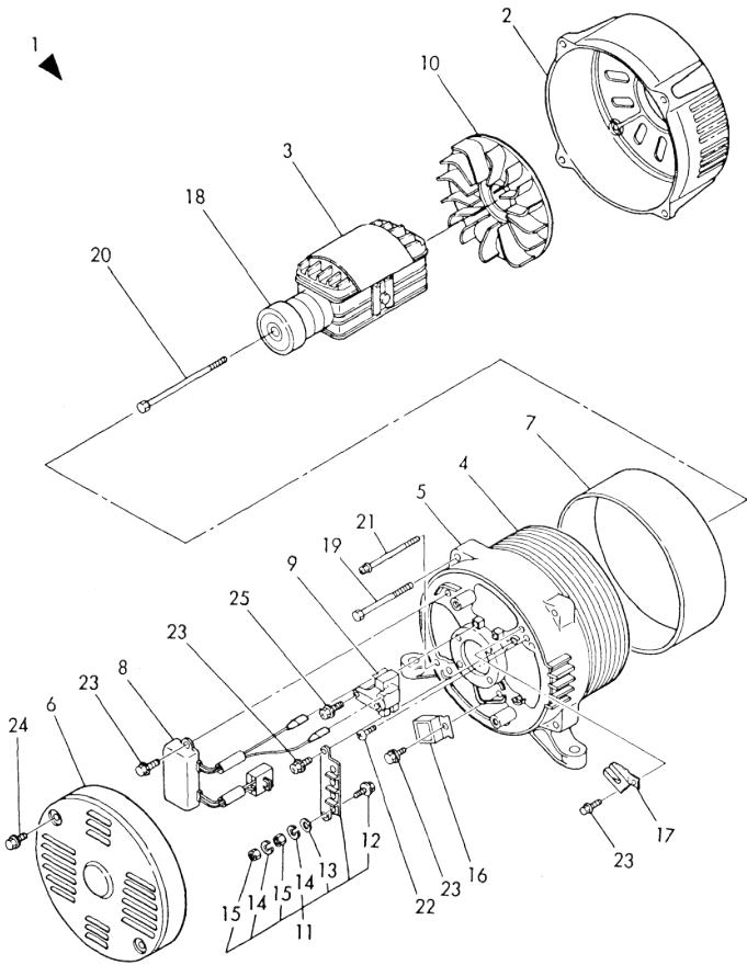
Fig. 29 GENERATOR
