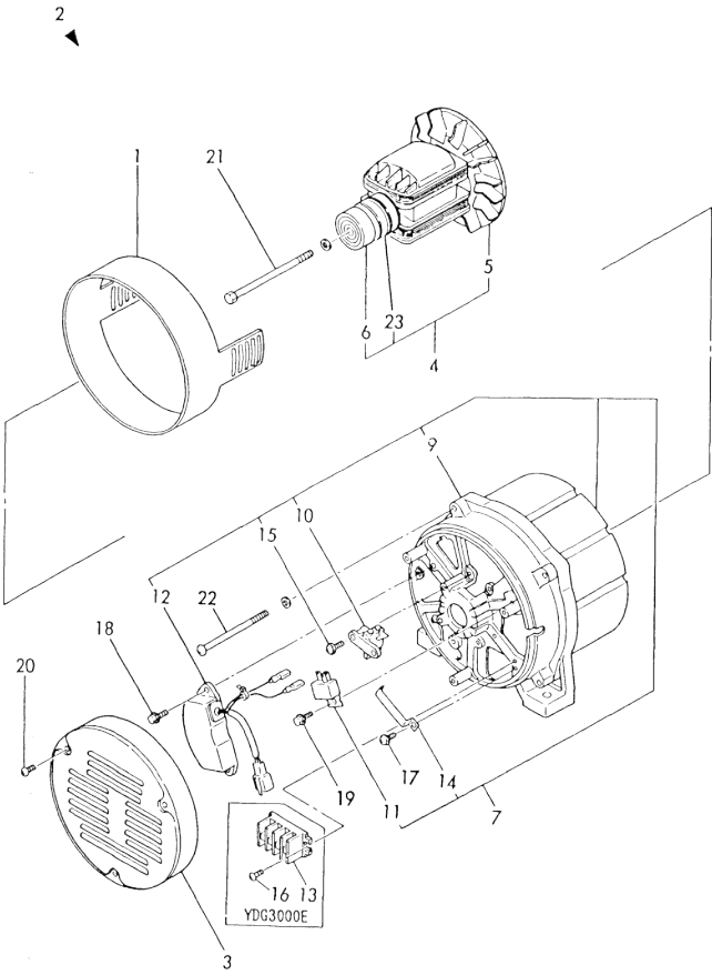
Fig. 103 GENERATOR
