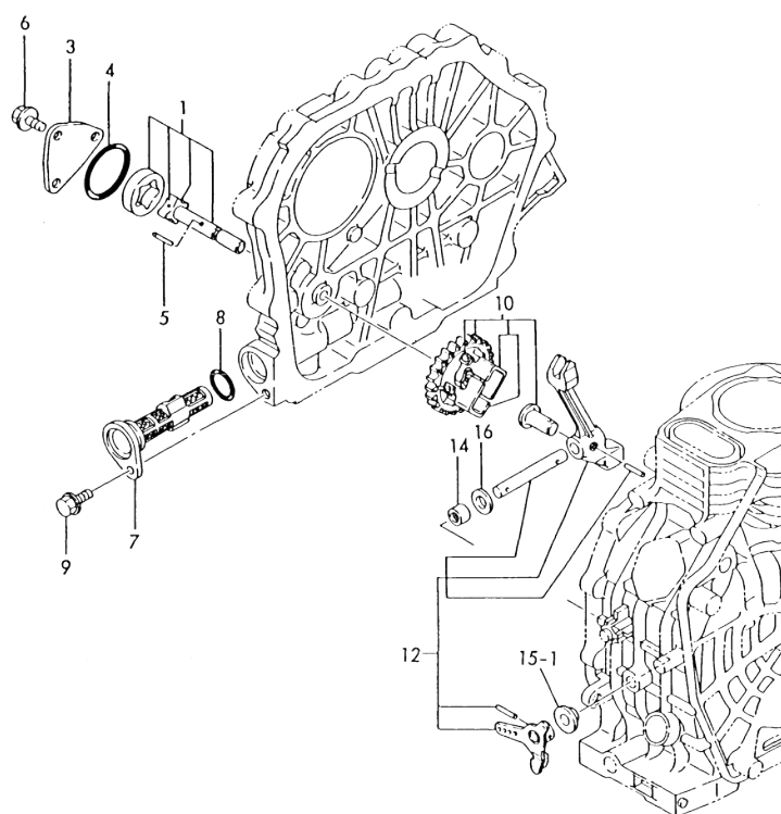
Fig. 111 L. O. DEVICE & GOVERNOR
