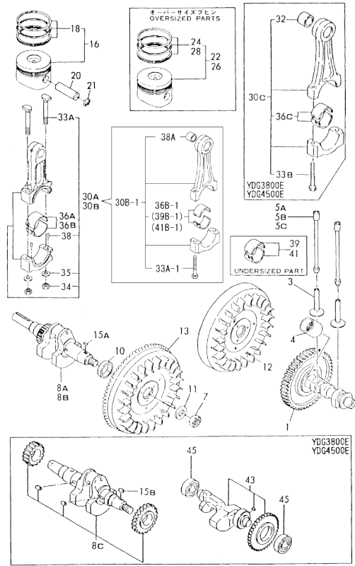
Fig. 19 CRANKSHAFT / PISTON / ROD
