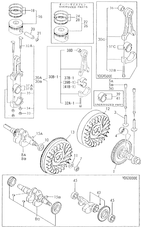
Fig. 35 CRANKSHAFT / PISTON / ROD
