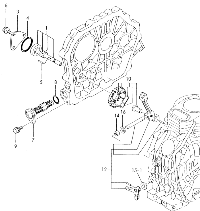
Fig. 20 L. O. DEVICE & GOVERNOR
