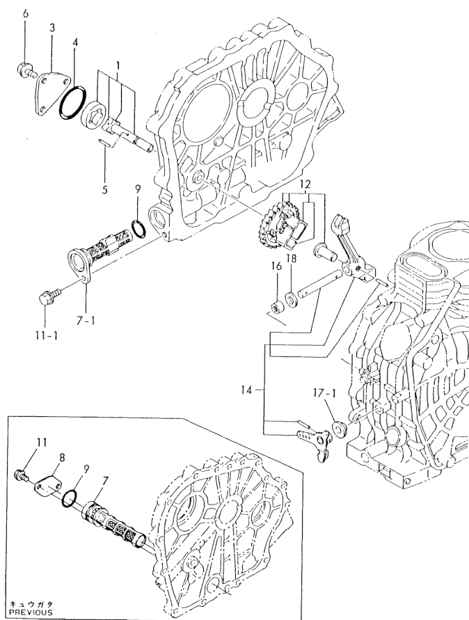
Fig. 82 L. O. DEVICE & GOVERNOR
