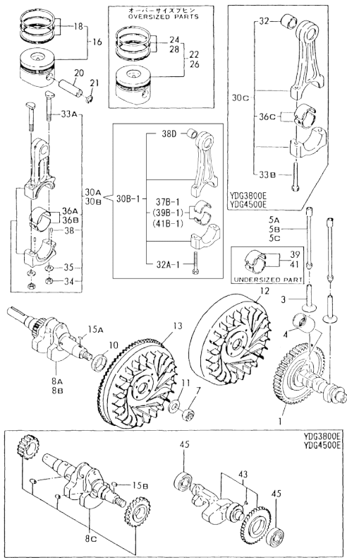
Fig. 110 CRANKSHAFT / PISTON / ROD
