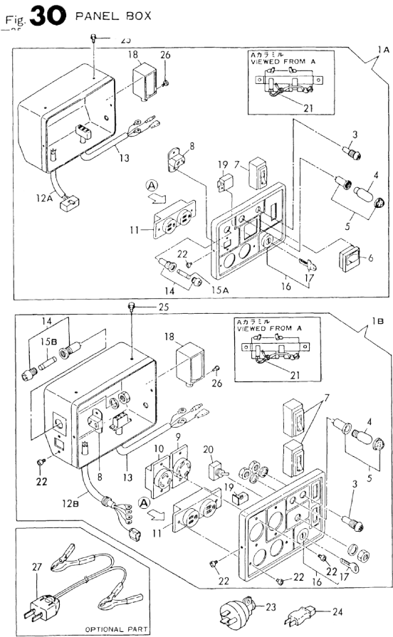
Fig.30. PANEL BOX (KOKUSAN-USA)
