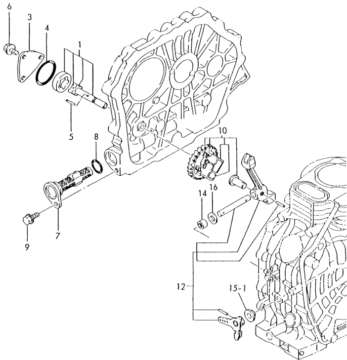
Fig.36 L. O. DEVICE & GOVERNOR
