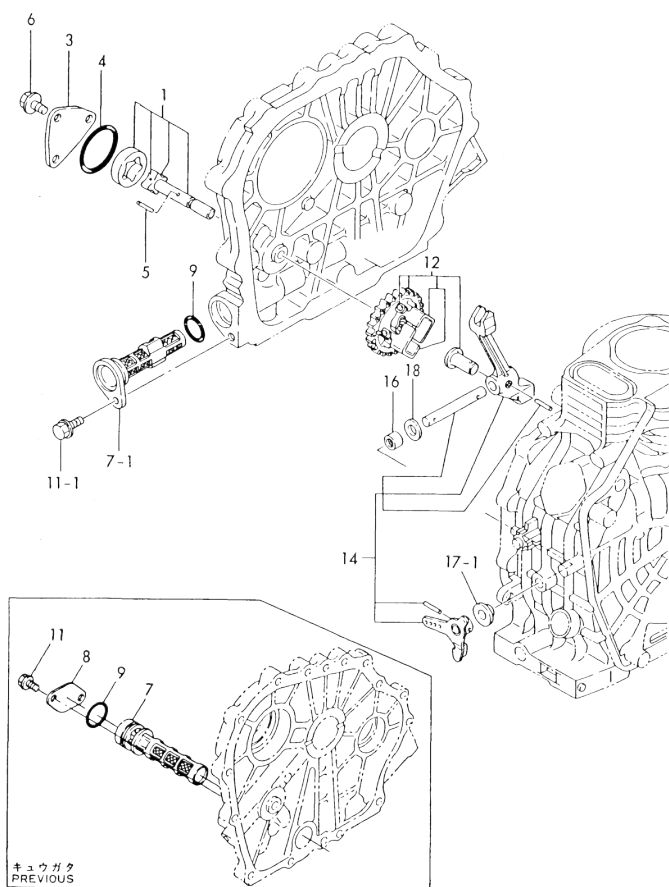
Fig. 5 L. O. DEVICE & GOVERNOR
