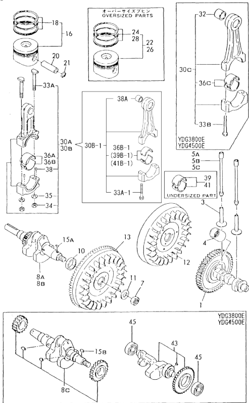
Fig. 94 CRANKSHAFT / PISTON / ROD
